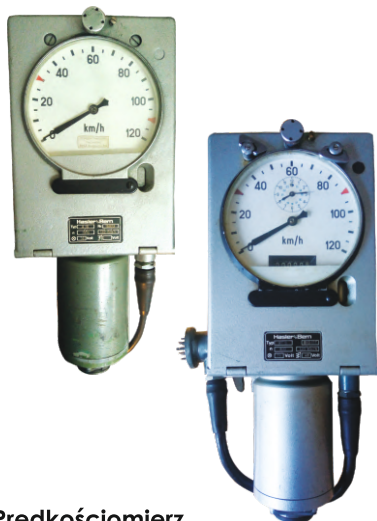
Prędkościomierz Hasler - Legalizacja Hasler speedometers - Legalization
