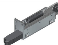
Rygiel dolny układu blokady drzwi DL-O 17 020-01
