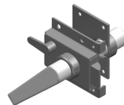
Zamek górny kabiny maszynisty zewnętrzny DL-O 17 062-03
